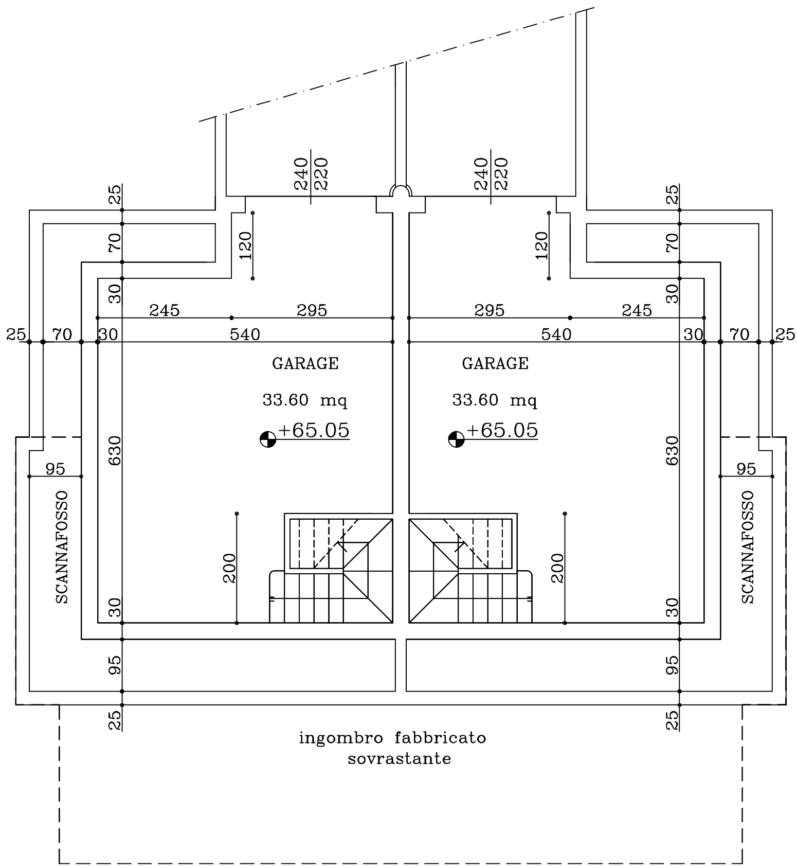
PIANTA PIANO INTERRATO
