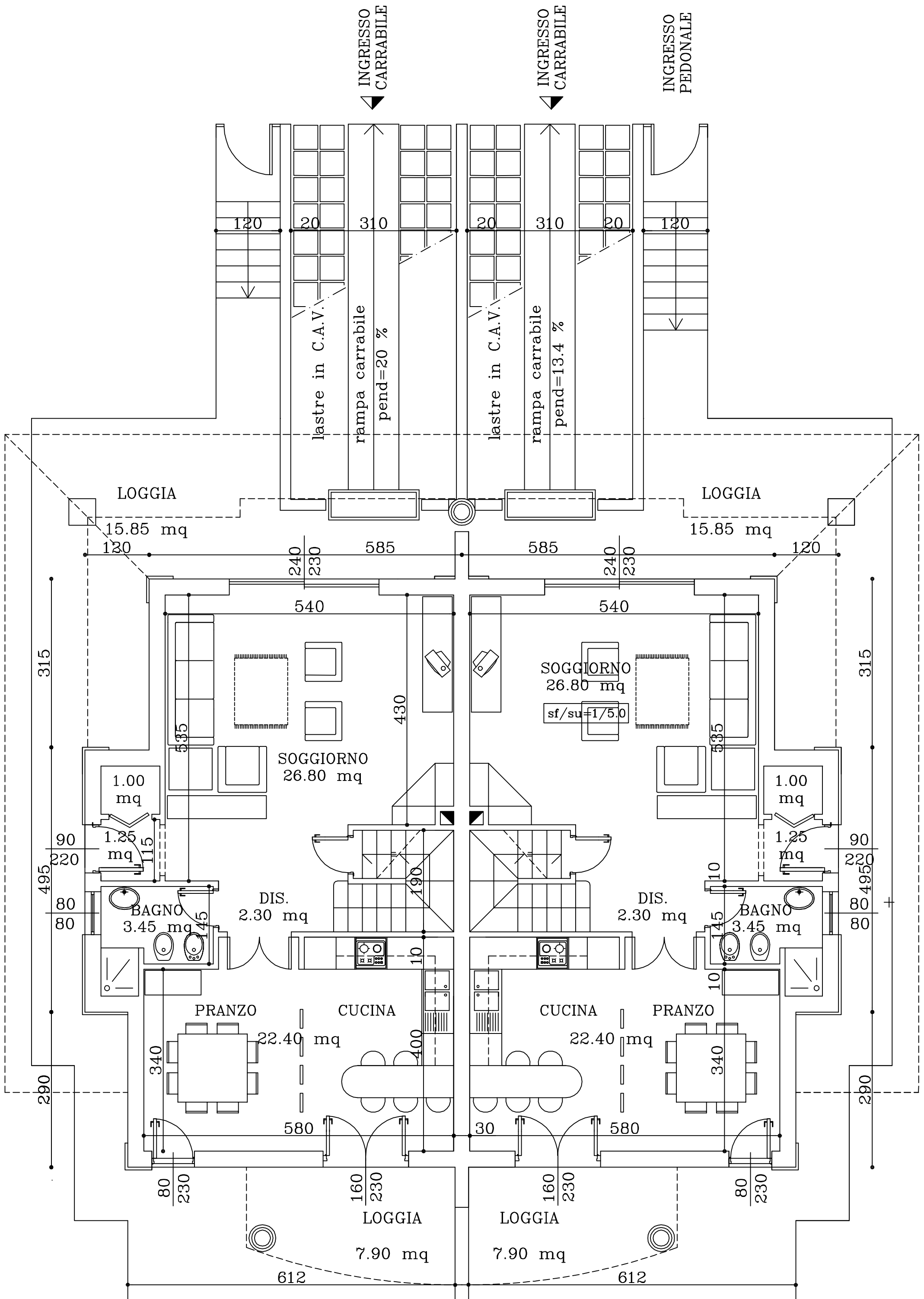
PIANTA PIANO TERRENO
